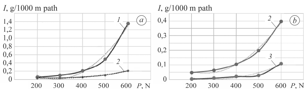
Рис. 1. Залежність інтенсивності зношування пар тертя під час сухого тертя від навантаження ( V = 2,25 m/s): a – пара сталь 20 (1)/сталь DDT 68 (2); b – сталь 45 (3)/сталь DDT 68 (2).
