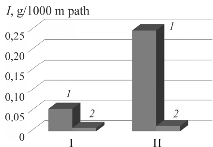
Рис. 2. Узагальнення досліджень в умовах сухого тертя (I – без наводнення; II – з наводненням ролика зі сталі DDT 68): 1 – сталь DDT 68; 2 – сталь 45 ( P = 250 N; V = 2,25 m/s).
