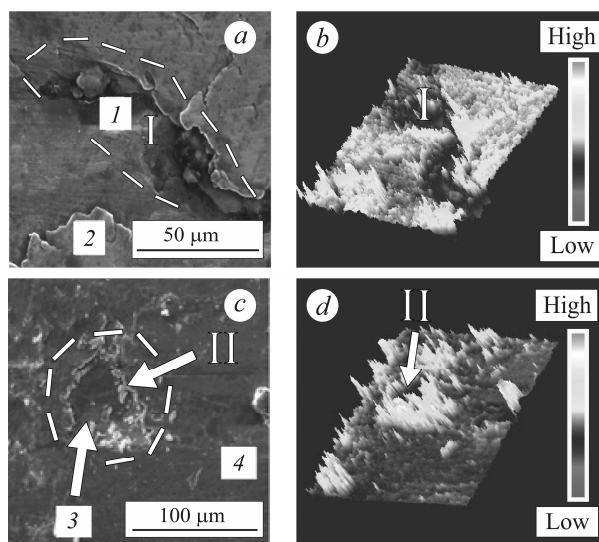
Рис. 5. Поверхня тертя з пошкодженням сталі 45 (a) та DDT 68 (c) та їх 3D реконструкція (b, d) (зона I, II відповідно): P = 500 \text{ N} ; V = 2,25 \text{ m/s} .
