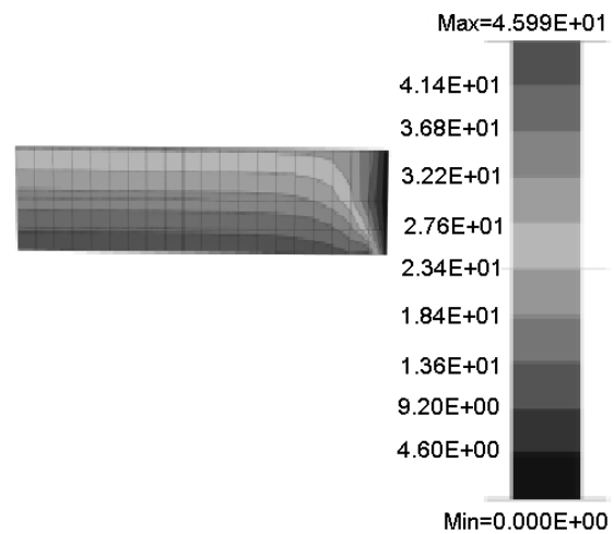
Рис. 2 - Розподіл температур \Delta T при сітці 4x21x21
