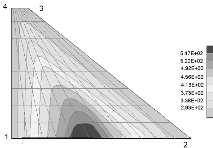
Рис. 3 - Розподіл температур на поверхні плити
