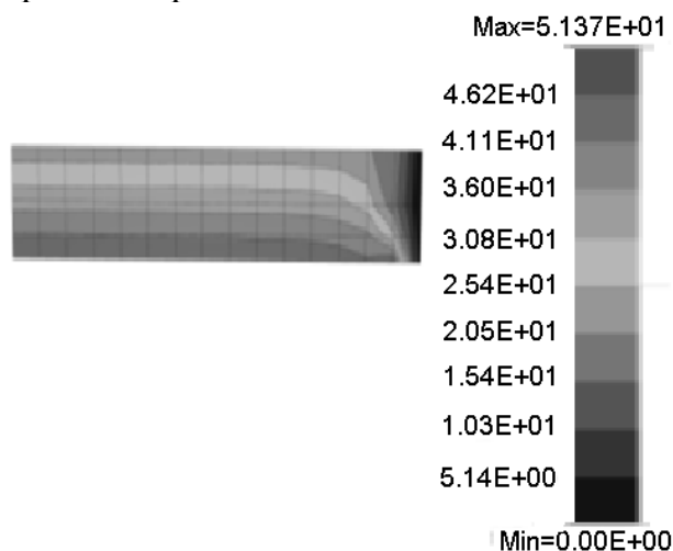
Рис. 1 - Розподіл температур \Delta T при сітці 4x16x16
