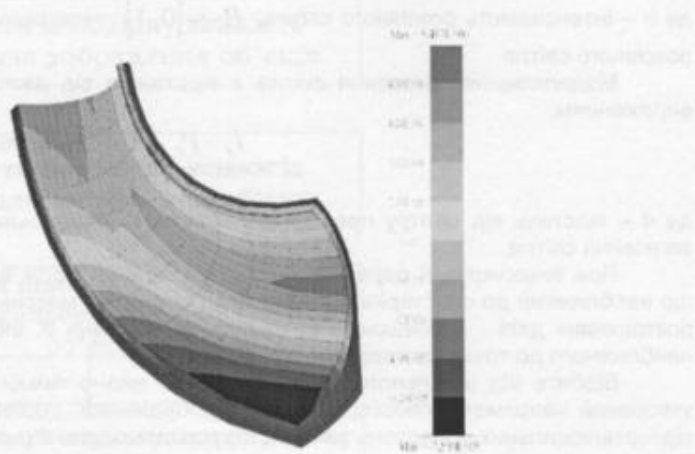
Рис. 7. Кольоровий розподіл \sigma_{yy}
