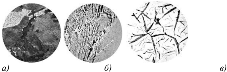
Рис. 7. Мікроструктури чавунів: а — Сірий чавун на перлитовій металевій основі. Крабовидні включення графіту (чорний) в перлитовій матриці. На стиках кордонів зерен перлиту видно світло-пестрі ділянки потрійної фосфідної евтектики. б — Ледебурит в евтектичному чавуні. Видно декілька колоній ледебуриту. в - Пластинчасті включення графіту. Структура металевісної основи не є показовою, оскільки шліф не труєний.
