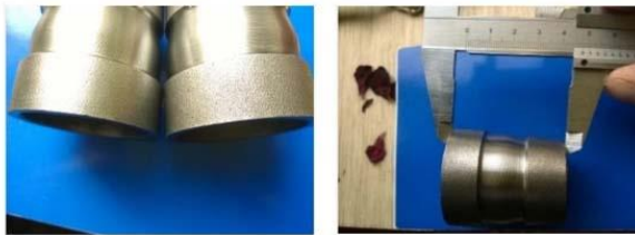
Рис. 6. Зліва – після вібрації, праворуч – нормальний знос (а); Розпірна втулка під час вимірювання (б)
