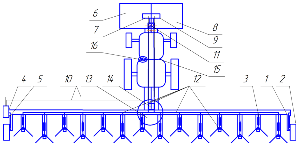
Рис. 1. Посівний агрегат (комплекс): 1 – рама; 2 – опорне колесо; 3 – змінні начіпні секції; 4 – блок керування; 5 – привід; 6, 8 – зерновий та туковий бункер; 7, 9 – дозатор; 10 – канали керування дозаторами; 11 – вентилятор; 12 – розподіляючі канали (зернотукопровід); 13 – бак для пестицидів; 14 – дозатор пестицидів; 15 – енергетичний засіб; 16 – бортовий комп'ютер
