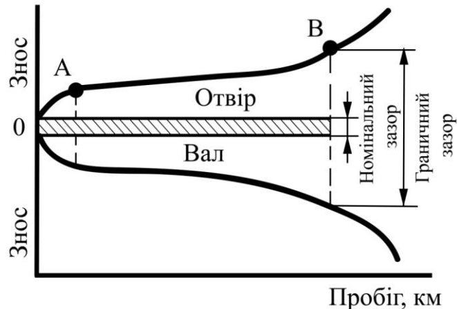
Рис. 2. Графік залежності зносу деталей від пробігу автомобіля [13]
