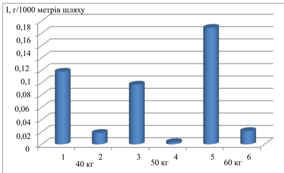
Рис.1. Експериментальні результати досліджень в умовах сухого тертя
